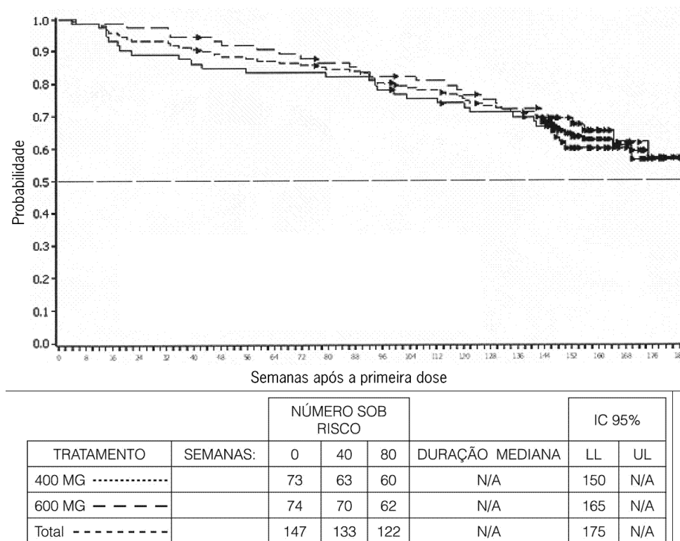
Figura 3: Estimativa Kaplan-Meier de sobrevida global desde o início do estudo por tratamento
